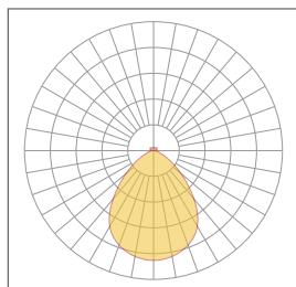
Symmetrical 85° H00200+H00220
