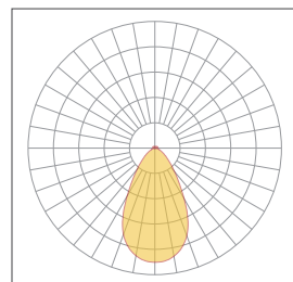
Symmetrical 60° H00200+H00221
