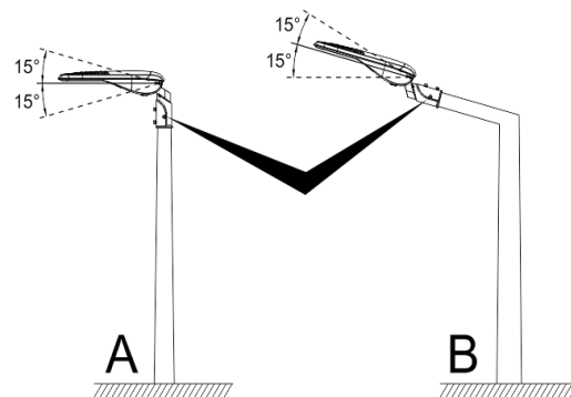
(Adjustable Angle)
